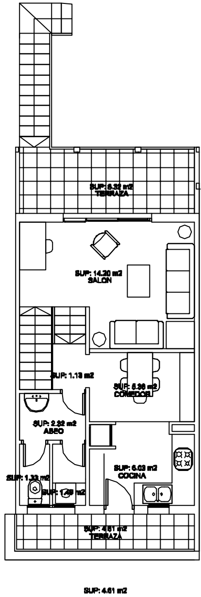
PLANTA ALTA
